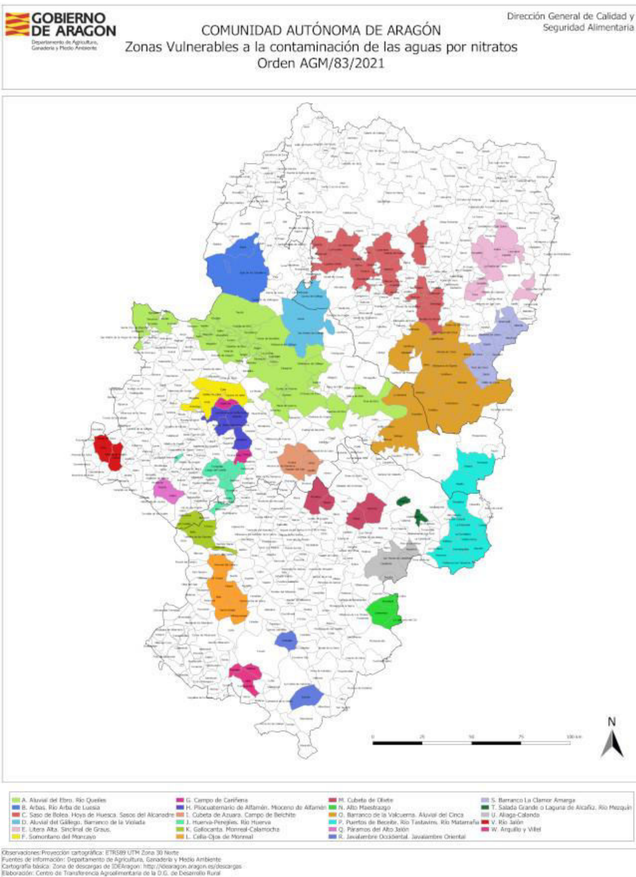
Ilustración 12: Mapa de zonas vulnerables a la contaminación por nitratos
