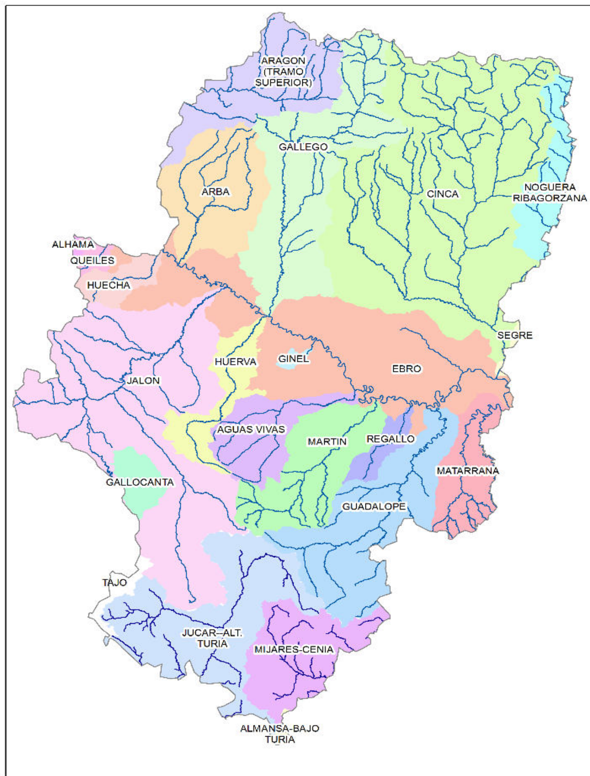
Ilustración 9: Cuencas hidrográficas en Aragón
