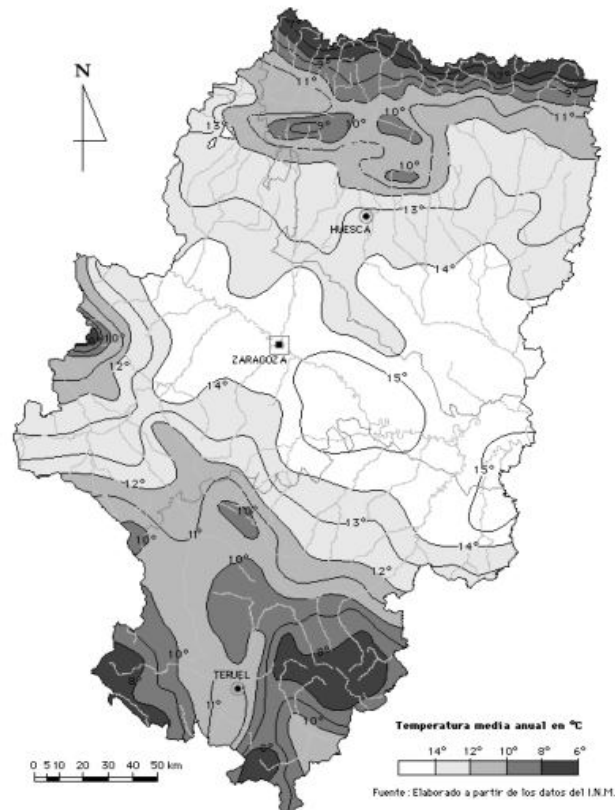
Ilustración 5: Mapa de isotermas medias anuales de Aragón
