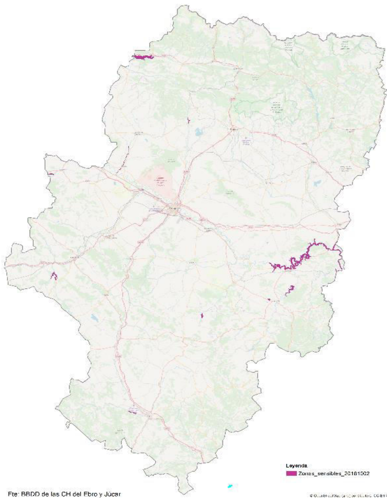
Ilustración 13: Mapa de zonas sensibles en Aragón
