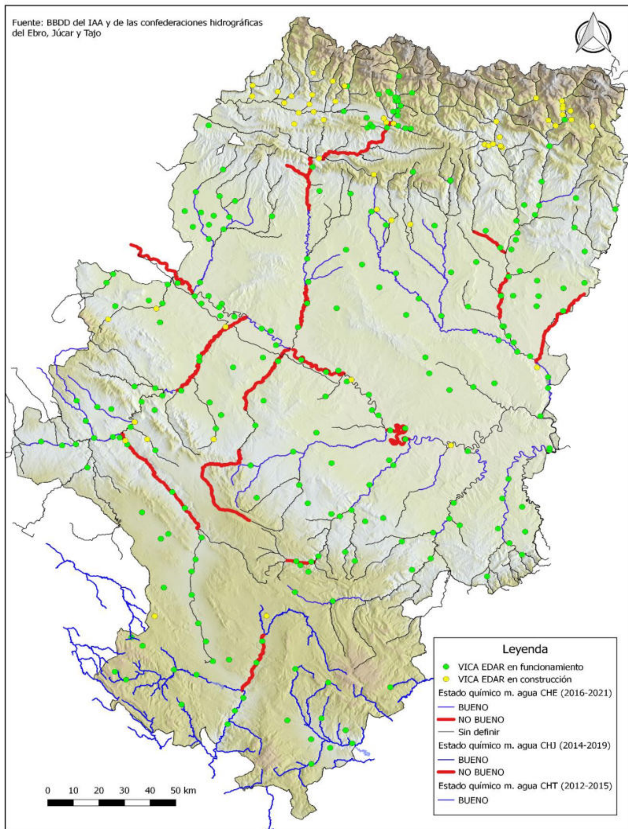
Ilustración 11: Estado químico de las masas de agua superficiales lineales
